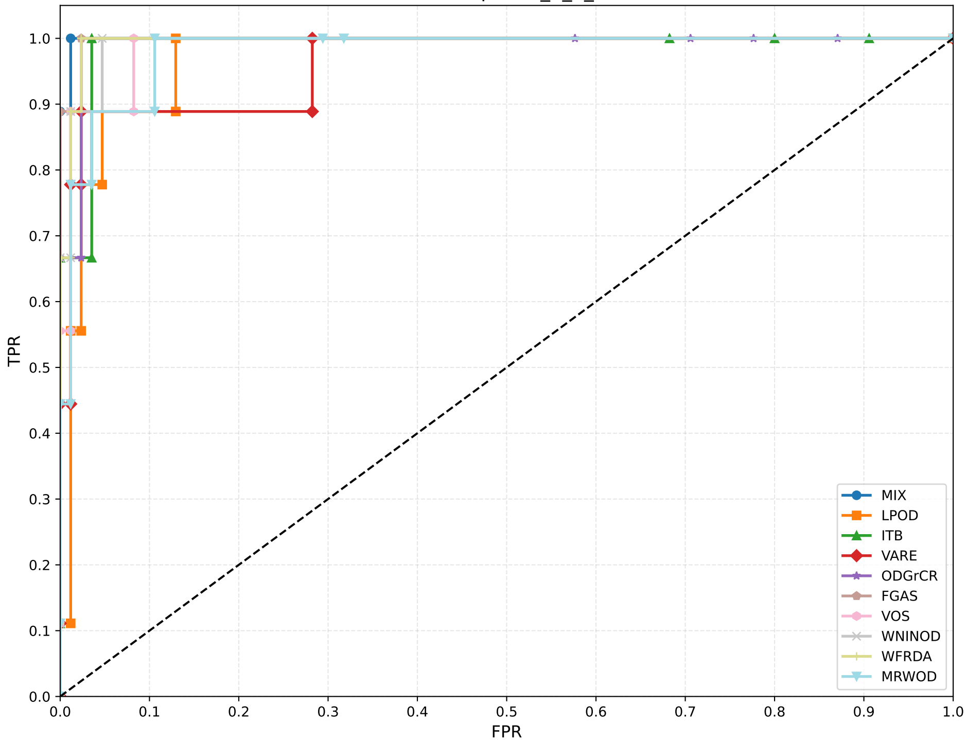
ROC Curve: hepatitis_2_9_variant1
