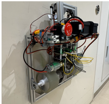
Fig. 2 スクレーパ機構を統合した実機外観
