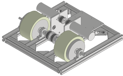
Fig. 1 開発した対向二輪式足回り機構
