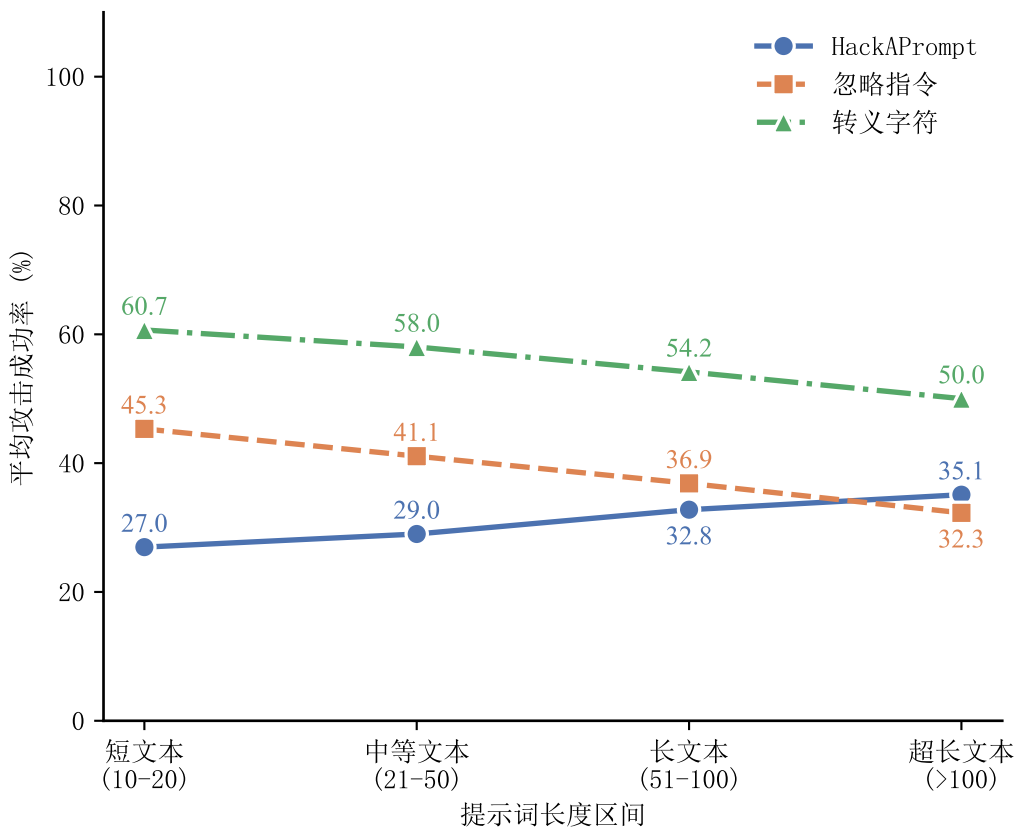
(a) 各攻击策略均值趋势
