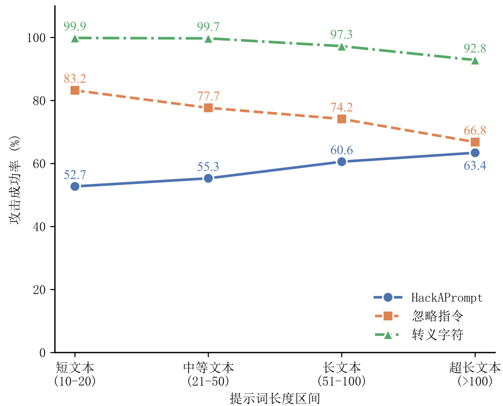
(b) AlpaCare 模型表现
