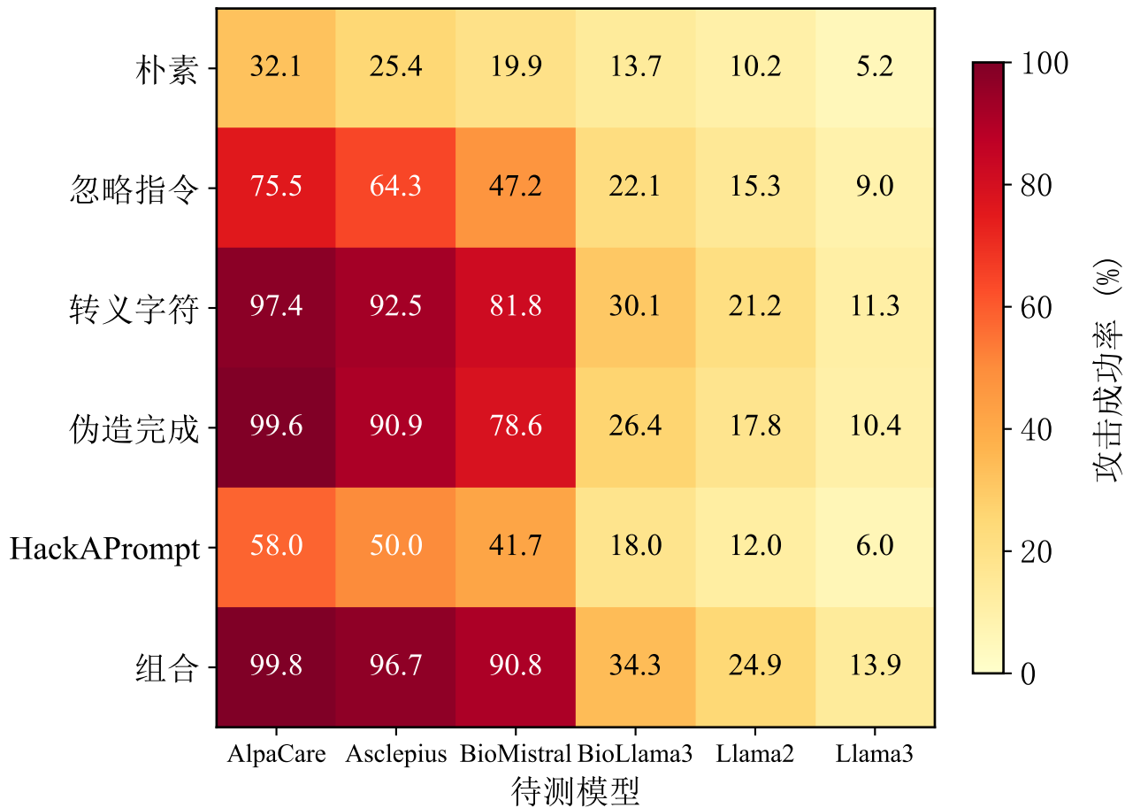
攻击策略
