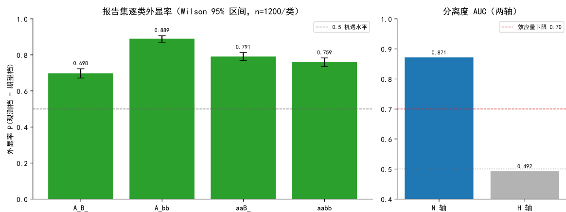
图 6: penetrance 报告集 (3 seed × 4 类 × 400, n = 1200 每类)。左: 逐类外显率及其 Wilson 95% 区间, 虚线为 0.5 机遇水平; 右: 两轴分离度 AUC, 红虚线为签署的效应量下限 0.70。N 轴可分离而 H 轴不可分离, 故生效轴取单轴 N。
