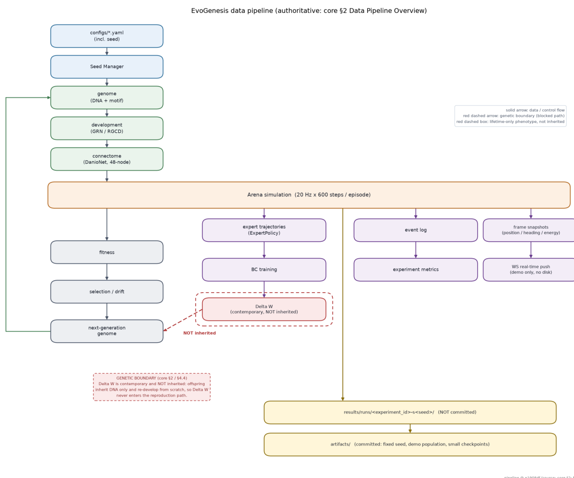
图 1: 整体数据流 (F12)。骨架为 configs (含 seed) → Seed Manager → genome (DNA + motif) → 发育 (GRN / RGCD) → 连接组 (DanioNet) → Arena (20 Hz × 600 步); Arena 之后分成三条并行同源分支: 专家轨迹 → BC 训练 → \Delta W 、事件日志 → 实验指标、帧快照 → WS 推送 (仅演示、不落盘); 再由 fitness → selection/drift 产生下一代 genome。红虚线框与红虚线边标出遗传边界: \Delta W 是当代的、不遗传, 后代只继承 DNA 并从发育重新开始。底部的 results/runs/ (不入库) 与 artifacts/ (入库) 是两个去向。节点与边的逐条出处 (core §2 等) 见同名.xlsx 的 nodes / edges 两个 sheet。
