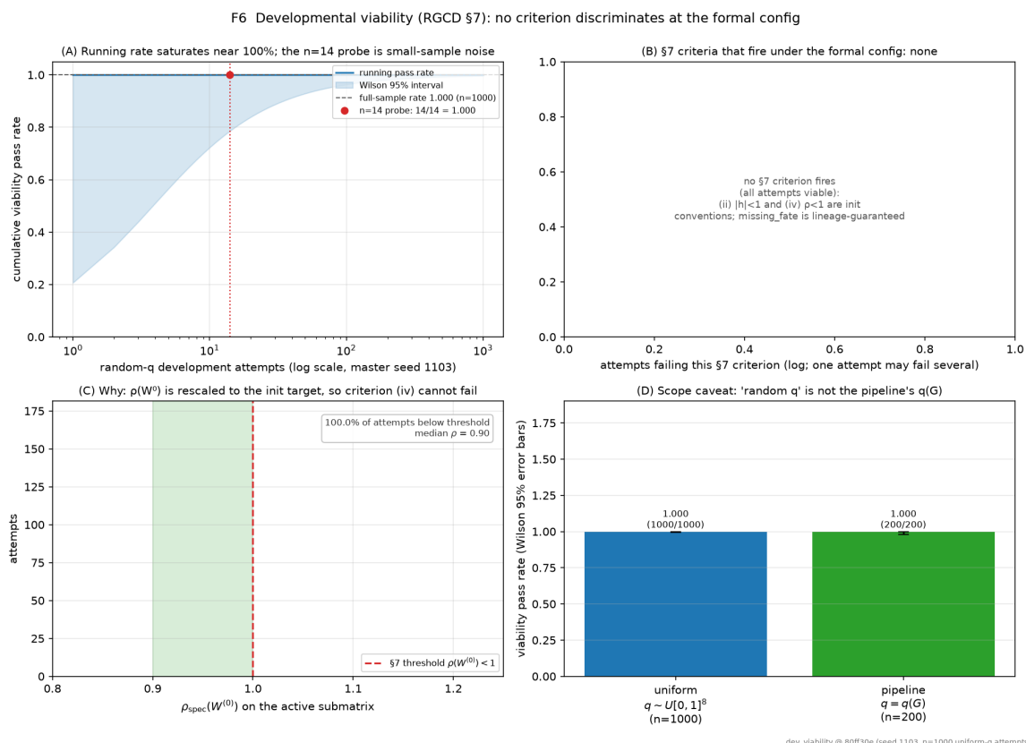
图 2: 发育 viability 通过率 (F6)。四个面板: (A) 累计通过率与 Wilson 区间, 标出 n = 14 冒烟点的位置; (B) 各判据的失败次数 (正式配置下为空: 无判据触发); (C) \rho(W^0) 分布与阈值 1.0 (已被重定到初始化目标, 故呈单点); (D) 随机 q 与 pipeline q(G) 的口径对照。本图的结论是无判据在筛人: 正式配置下 1000 次随机 q 全部通过 ( 1000/1000 = 100\% , Wilson [99.6\%, 100.0\%] ), pipeline q(G) 口径 200/200, 八项判据零次触发。原因是判据 (ii) |h| < 1 (解析保证)、判据 (iv) \rho(W^0) < 1 (初始化重定保证) 与 missing_fate ( c_{\text{domain}} 谱系先验保证) 三者均为设计约定, 恒真而不贡献区分力。故不得据本图宣称发育是强约束筛选; 筛选压力归代际适应度 F 。解除三处约定可复现旧读数 (4.7% 通过、 \rho 占 92% 拒绝), 但该读数由失配阈值主导、可绑定区是致死的逐 seed 彩券, 标定扫描见 research/notes/契约决策记录.md 。数据与复现命令见同名.xlsx 的 _manifest。
