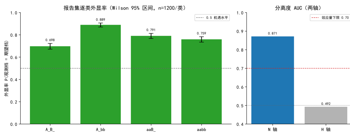
图 6: penetrance 报告集 (3 seed × 4 类 × 400, n = 1200 每类)。左: 逐类外显率及其 Wilson 95% 区间, 虚线为 0.5 机遇水平; 右: 两轴分离度 AUC, 红虚线为签署的效应量下限 0.70。N 轴可分离而 H 轴不可分离, 故生效轴取单轴 N。
