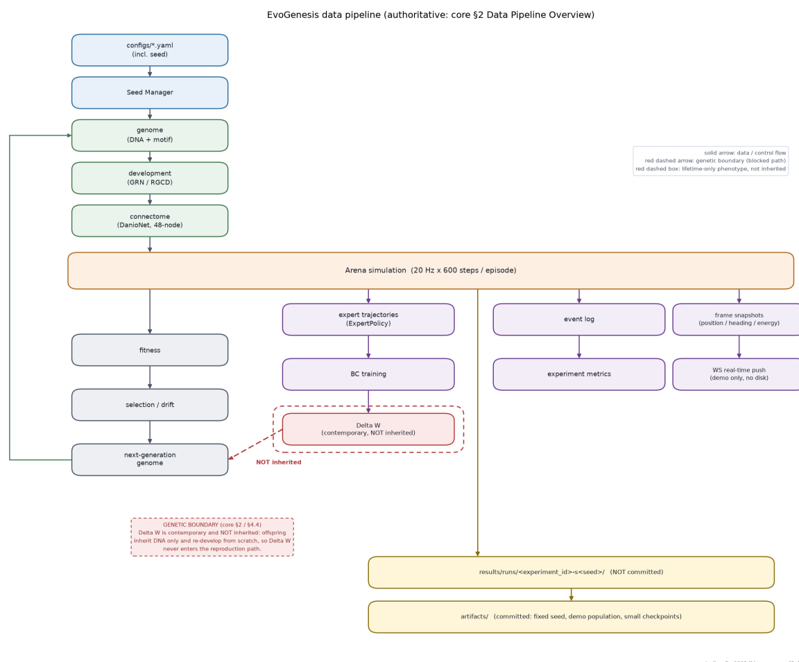
图 1: 整体数据流 (F12)。骨架为 configs (含 seed)、Seed Manager、genome (DNA 与 motif)、发育 (GRN / RGCD)、连接组 (DanioNet)、Arena (20 Hz × 600 步); Arena 之后分成三条并行同源分支: 专家轨迹、BC 训练、 \Delta W 、事件日志、实验指标、帧快照、WS 推送 (仅演示、不落盘); 再由 fitness、selection/drift 产生下一代 genome。红虚线框与红虚线边标出遗传边界: \Delta W 是当代的、不遗传, 后代只继承 DNA 并从发育重新开始。底部的 results/runs/ (不入库) 与 artifacts/ (入库) 是两个去向。节点与边的逐条出处 (core §2 等) 见同名.xlsx 的 nodes / edges 两个 sheet。
