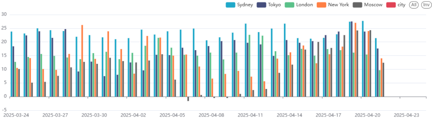
weather_data_bar_chart
