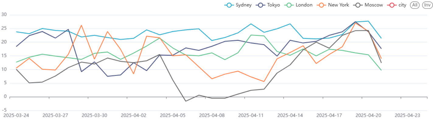
weather_data_line_chart
