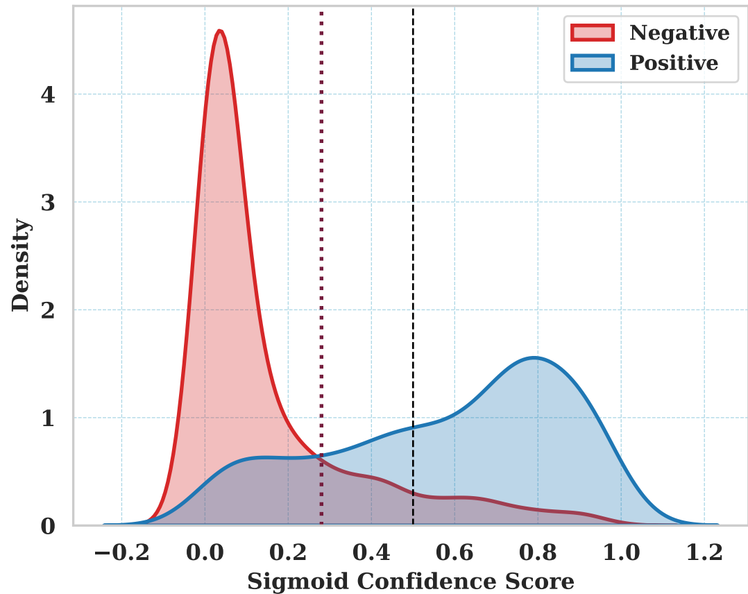
KDE Plot: Effusion
