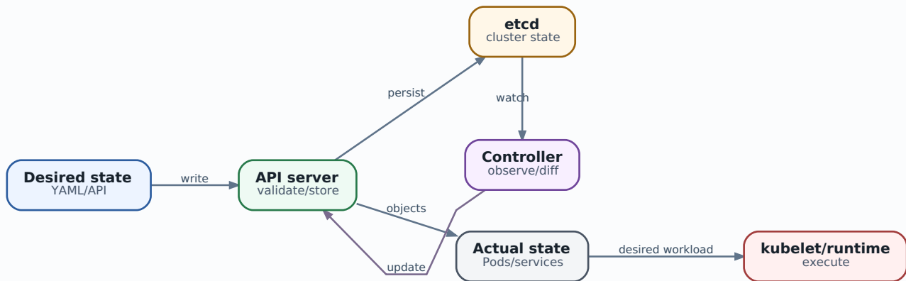
Kubernetes reconciliation loop - mental model, который нужен для AX/Substrate
