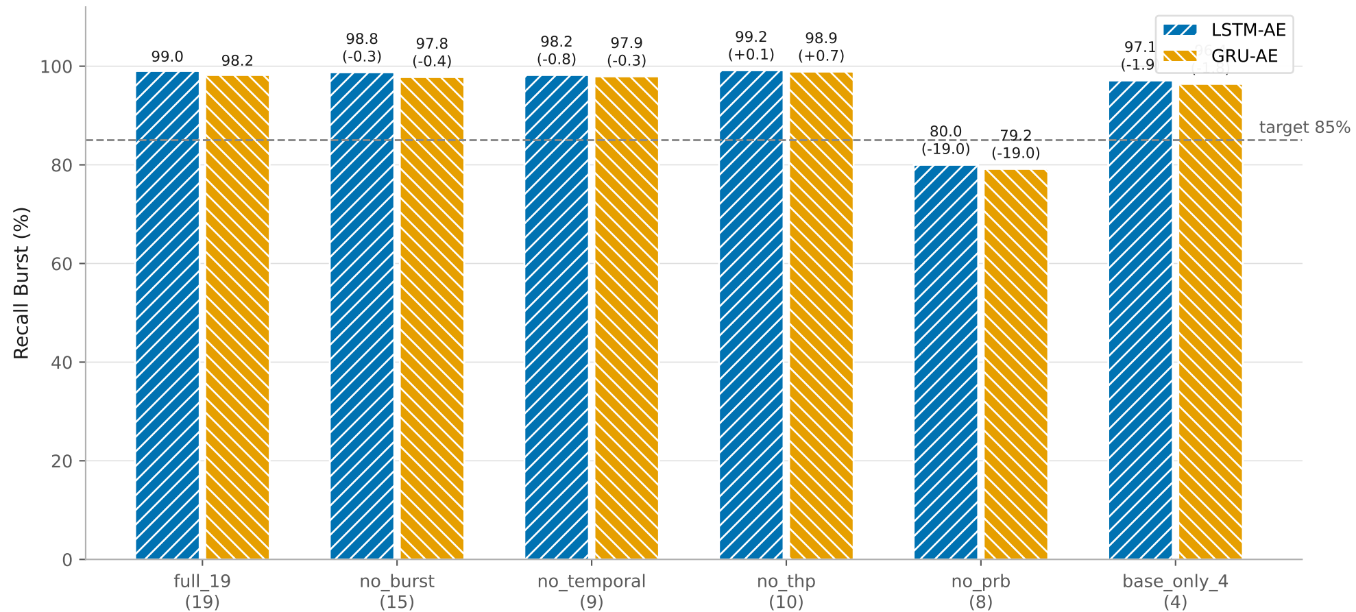
Penurunan Recall Burst setelah Kelompok Fitur Dihapus — ML-Only, seed 42
