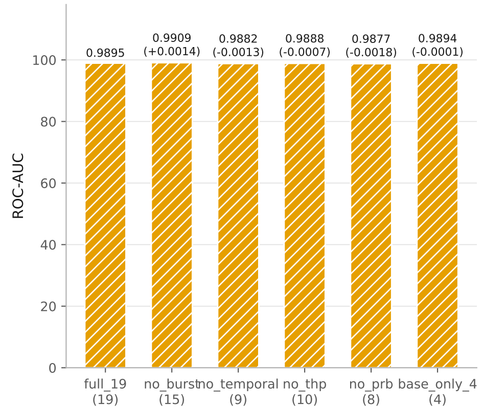
ROC-AUC
