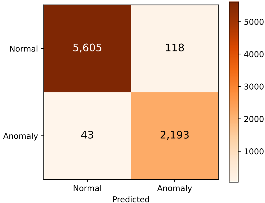
GRU-HYBRID
