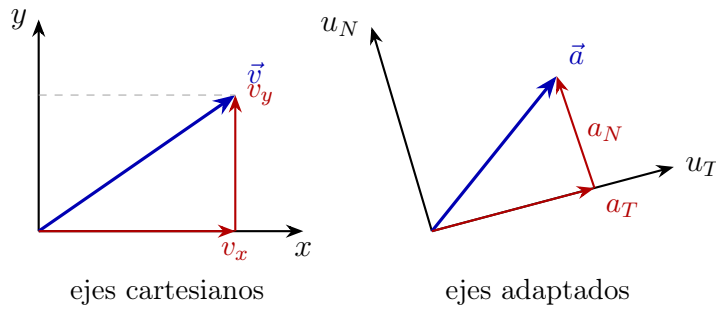
Figura 10: Descomposición vectorial en componentes perpendiculares.
