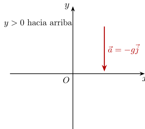
Figura 8: Sistema de referencia para la caída vertical.
