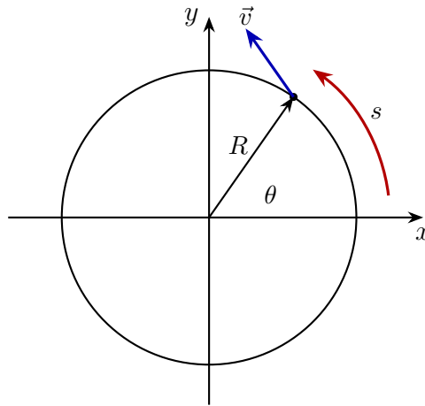
Figura 15: Representación de un movimiento circular.
