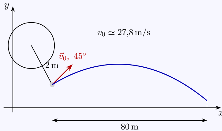
Figura 17: Lanzamiento con cuerda para alcanzar ochenta metros.
