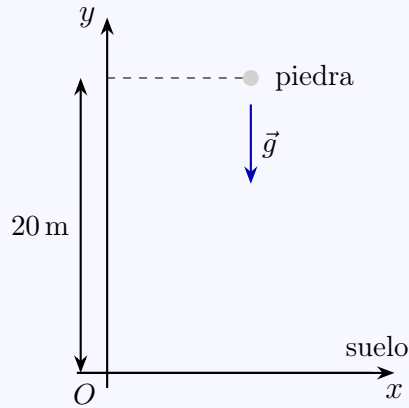
Figura 9: Esquema de la caída de una piedra desde veinte metros.
