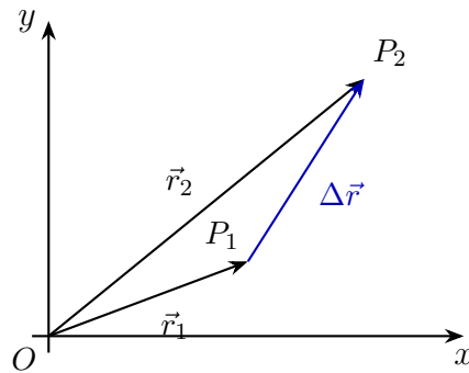
Figura 1: Representación del vector posición y el desplazamiento.
