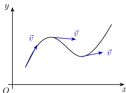
Figura 2: Vector velocidad tangente a la trayectoria.
