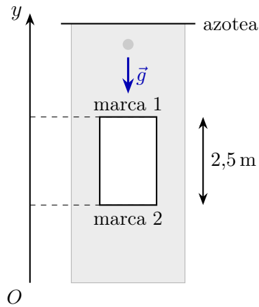
Figura 19: Caída de una bola al pasar por una ventana.
