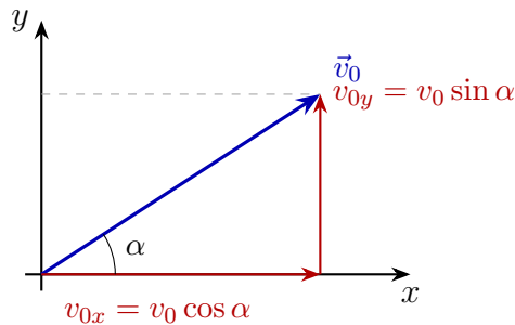
Figura 12: Componentes de la velocidad inicial en un lanzamiento.
