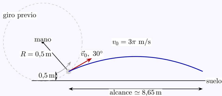
Figura 16: Salida parabólica de una piedra atada a una cuerda.
