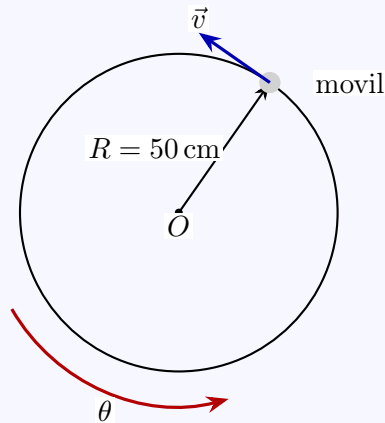
Figura 18: Móvil sobre una circunferencia de cincuenta centímetros.
