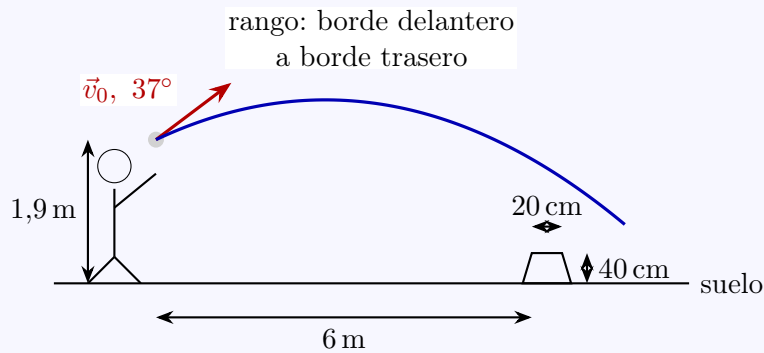
Figura 20: Lanzamiento parabólico hacia una papelera.
