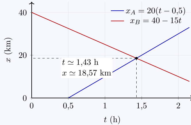
Figura 6: Gráfica posición-tiempo del encuentro.
