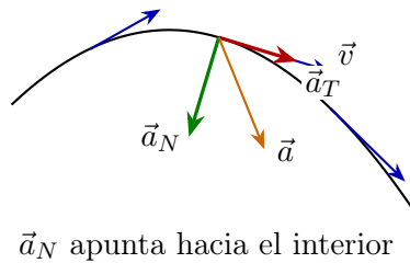
Figura 11: Componentes tangencial y normal de la aceleración.
