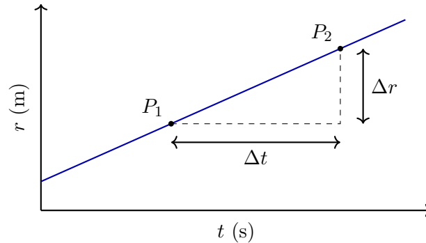
Figura 4: Gráfica posición-tiempo de un movimiento rectilíneo uniforme.
