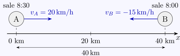
Figura 5: Esquema de encuentro entre dos móviles.
