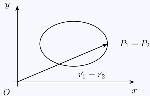
Figura 3: Trayectoria cerrada en un circuito.
