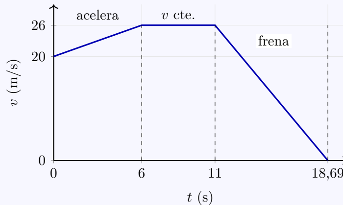
Figura 7: Gráfica velocidad-tiempo de un movimiento acelerado y frenado.
