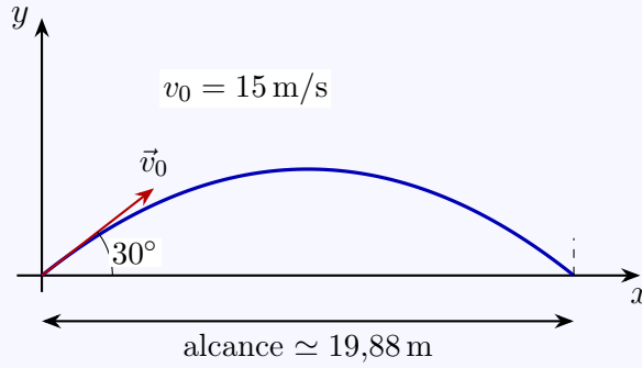
Figura 13: Lanzamiento parabólico con ángulo de treinta grados.
