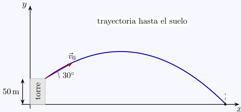
Figura 14: Lanzamiento parabólico desde una torre.
