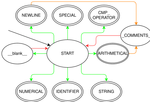
Obrázek: Abstrakce konečného stavového automatu lexéru
