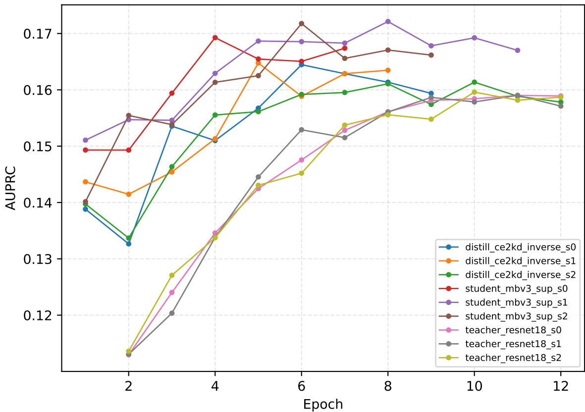
Val AUPRC
