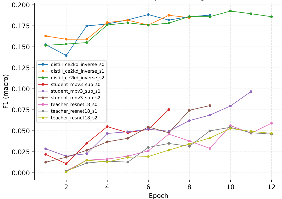
Val F1 (macro, per-class th@val)
