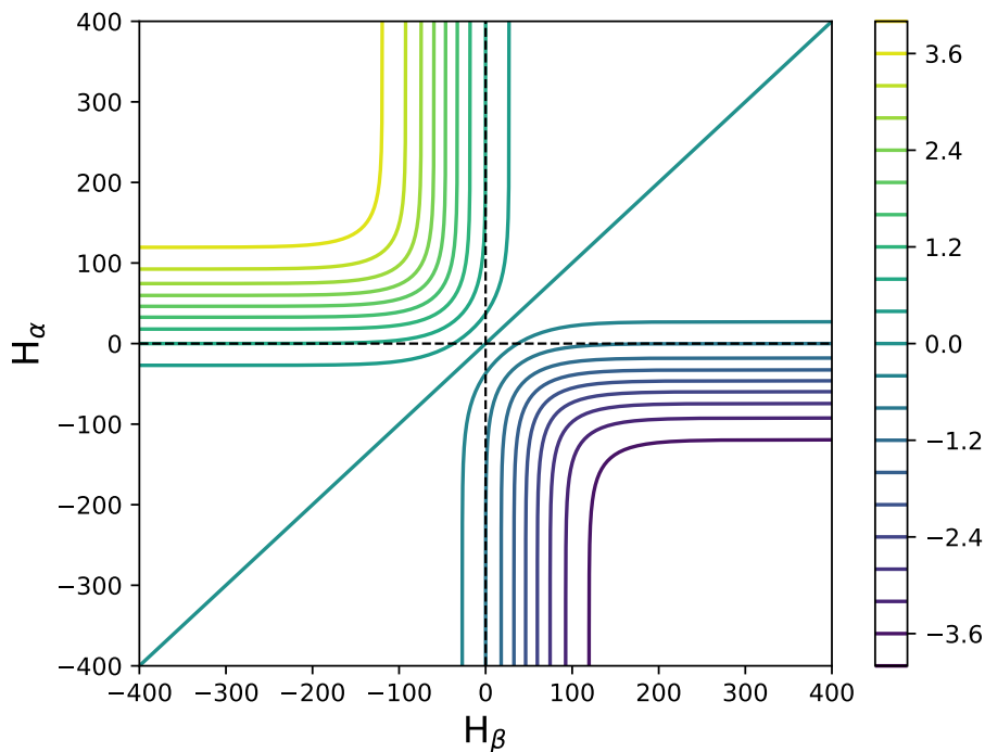
Slika 4.3: Funkcija (4.48) za parametre c = 1 , d = 0.25 i k = 0.03 . Restrikcija ove funkcije na područje iznad pravca H_\alpha \geq H_\beta predstavlja Everettovu funkciju
