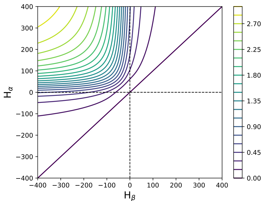
Slika 4.4: Everetova funkcija bazirana na funkciji (4.49) za parametre a = 0.0196483 , b = 2.95329554 , c = 0.02211744 , d = 1.04359946 i k = 0.1
