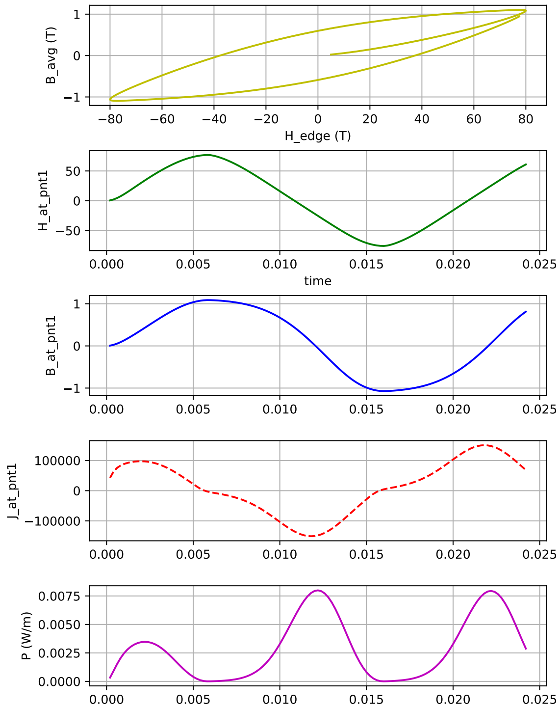
Slika 4.9: Reultati simulacije za problem vrtložnih struja u jednoj feromagnetskoj lameli s histereznim značajkama materijala. Prvi subplot pokazuje 1,2 vremenske periode petlje histereze za promatranu lamelu. Histereza je bazirana na Everettovoj funkciji (4.47). Drugi subplot pokazuje H(t) funkciju za jednu točku unutar lamele. Treći subplot pokazuje B(t) funkciju za istu točku unutar lamele. Isto tako, četvrti subplot pokazuje J(t) funkciju za tu točku unutar lamele. Na kraju, peti subplot pokazuje vremensku ovisnost ukupnih gubitaka u lameli o vremenu.
