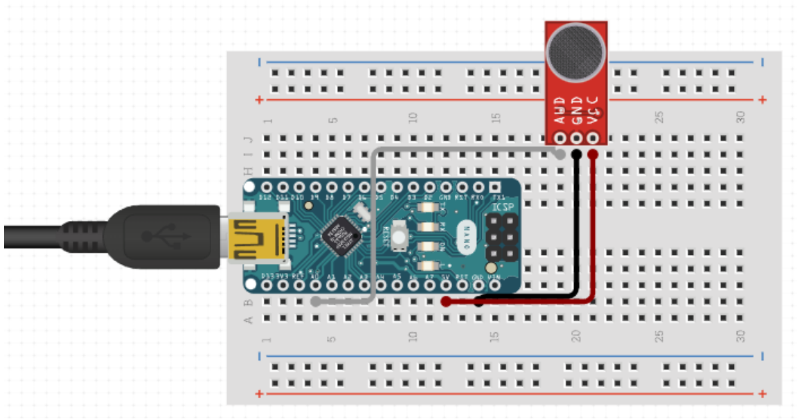
Рис. 1: Подключение модуля KY-037 к плате Arduino: выход АО модуля соединён с аналоговым входом АЦП, питание — от шины платы
