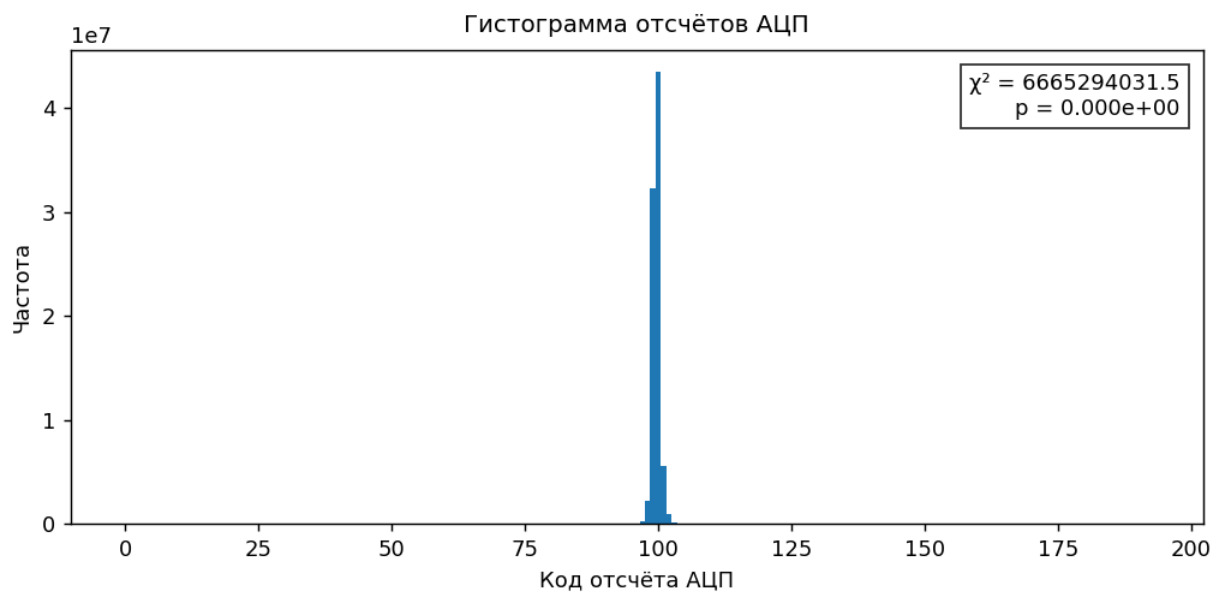
Рис. 2: Гистограмма распределения отсчётов АЦП для акустического канала
