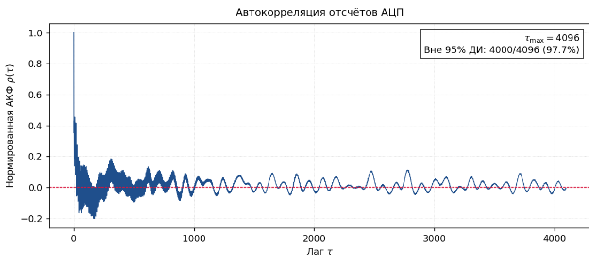
Рис. 3: Автокорреляция отсчётов АЦП (временная зависимость)
