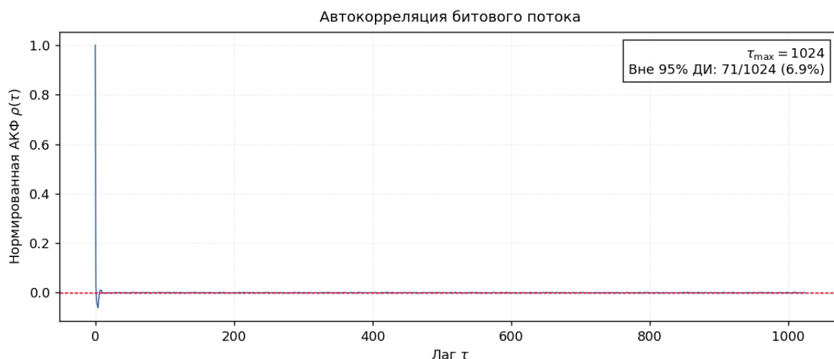
Рис. 6: Автокорреляция битового потока после постобработки по схеме фон Неймана
