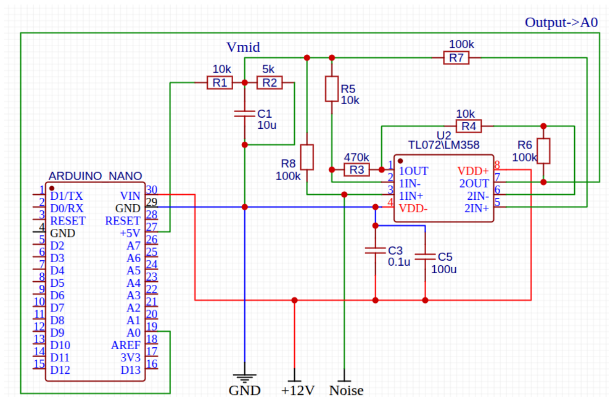
Рис. 2: Принципиальная схема двухкаскадного неинвертирующего усилителя на сдвоенном ОУ LM358 / TL072 при однополярном питании +12 В: R_1, R_2 — делитель V_{mid} (на схеме R_2 = 5 кОм, что соответствует скорректированному значению из раздела 3.5.4; в исходной конфигурации R_2 = 10 кОм); R_5, R_3 — цепь обратной связи первого каскада; R_4 — резистивная связь между каскадами; R_6 — обратная связь второго каскада; R_7 — резистор смещения неинвертирующего входа 2IN+ (пин 5) к шине V_{mid} . Выход 2OUT подаётся напрямую на вход АЦП A0 Arduino Nano
