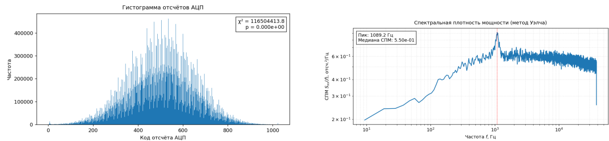
Рис. 9: Финальная конфигурация (этап 4): гистограмма и оценка спектральной плотности мощности. Распределение симметрично, спектр близок к плоскому в рабочей полосе
