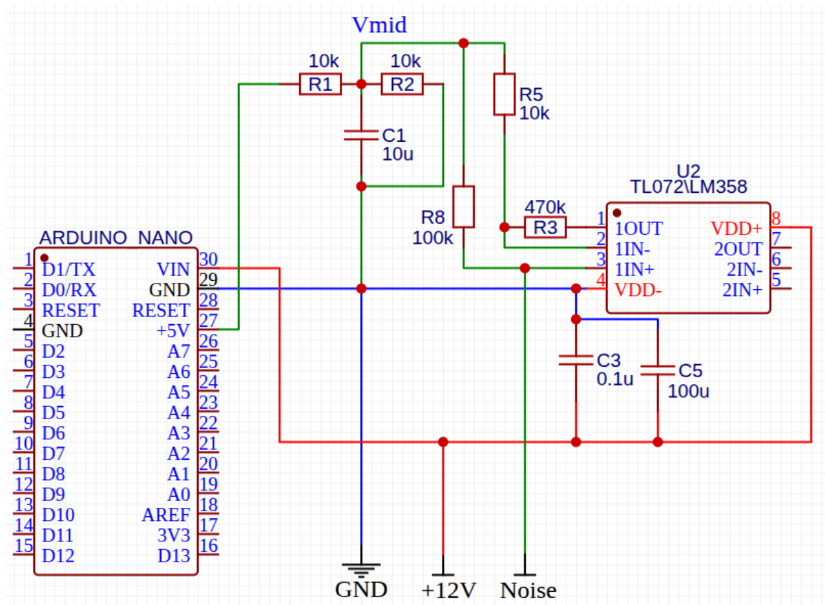
Рис. 1: Принципиальная схема однокаскадного неинвертирующего усилителя на ОУ LM358 / TL072 при однополярном питании +12 В: R_1, R_2 образуют делитель опоры V_{mid} , C_1 = 10 \text{ мкФ} — развязка опоры, R_5 = R_g и R_3 = R_f — цепь обратной связи, R_8 = 100 \text{ кОм} — входной согласующий резистор; C_3 = 0,1 \text{ мкФ} и C_5 = 100 \text{ мкФ} — развязка по питанию. Выход 1OUT подаётся на вход АЦП A0 Arduino Nano
