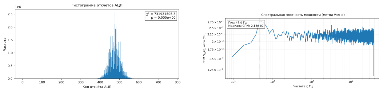
Рис. 6: Этап 1 (одиночный каскад): гистограмма отсчётов АЦП и оценка спектральной плотности мощности
