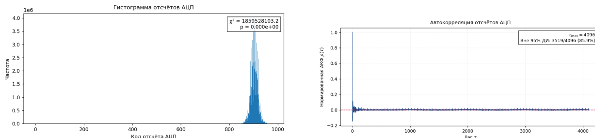
Рис. 4: Тепловой канал: гистограмма отсчётов АЦП ( N = 85 \cdot 10^6 ) и нормированная автокорреляция отсчётов
