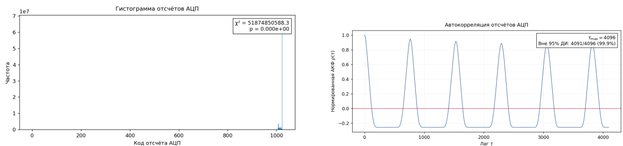
Рис. 13: Плавающий вход АЦП: гистограмма (концентрация в области \sim 1020 ) и автокорреляция отсчётов
