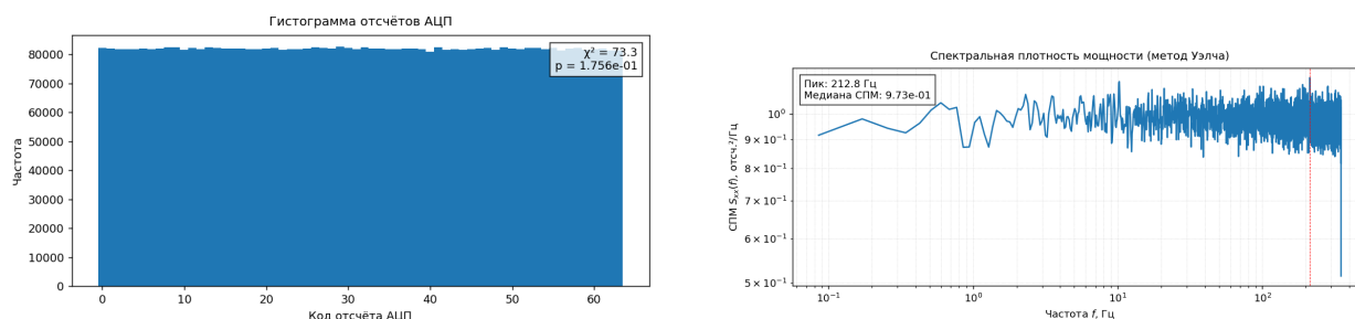
Рис. 14: MPU-6050: гистограмма выходных байтов и оценка спектральной плотности мощности
