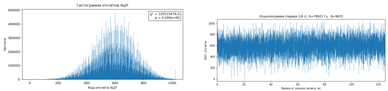
Рис. 7: Этап 2 (двухкаскадный усилитель): гистограмма отсчётов АЦП и осциллограмма первых 125 мс записи. На гистограмме видна выраженная аномалия — накопление отсчётов на верхней границе шкалы (значение 1023); на осциллограмме заметно «упирание» сигнала в потолок
