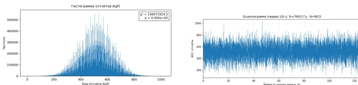
Рис. 8: Этап 3 (коррекция V_{\text{mid}} ): гистограмма стала практически симметричной, на осциллограмме «упираия» в потолок более не наблюдается
