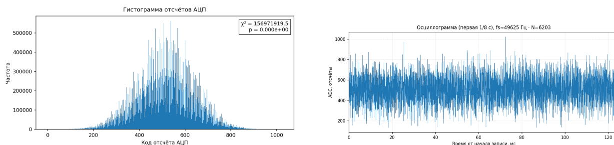
Рисунок 16 — Этап 3 (коррекция V_{\text{mid}} ): гистограмма стала практически симметричной, на оциллограмме «упирания» в потолок более не наблюдается
