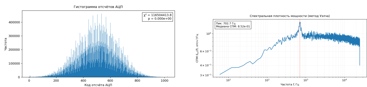
Рисунок 17 — Финальная конфигурация (этап 4): гистограмма и оценка спектральной плотности мощности. Распределение симметрично, спектр близок к плоскому в рабочей полосе
