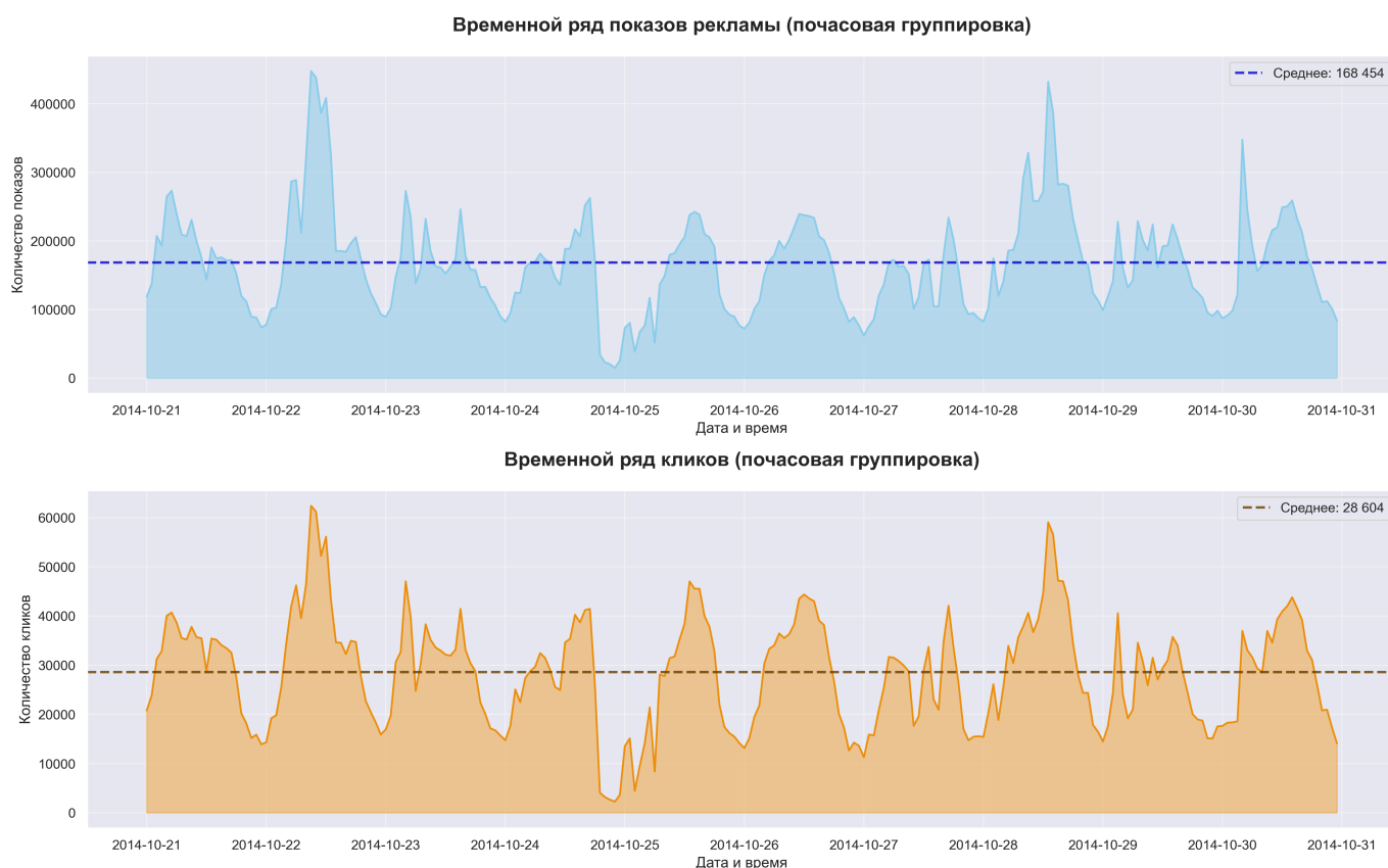
Рисунок 3.5. Временной ряд показов и кликов рекламы, почасовая группировка
