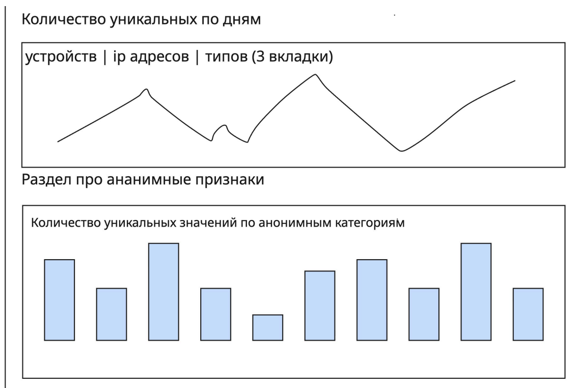
Рисунок 5.12. Динамика количества уникальных значений и анализ анонимных признаков
