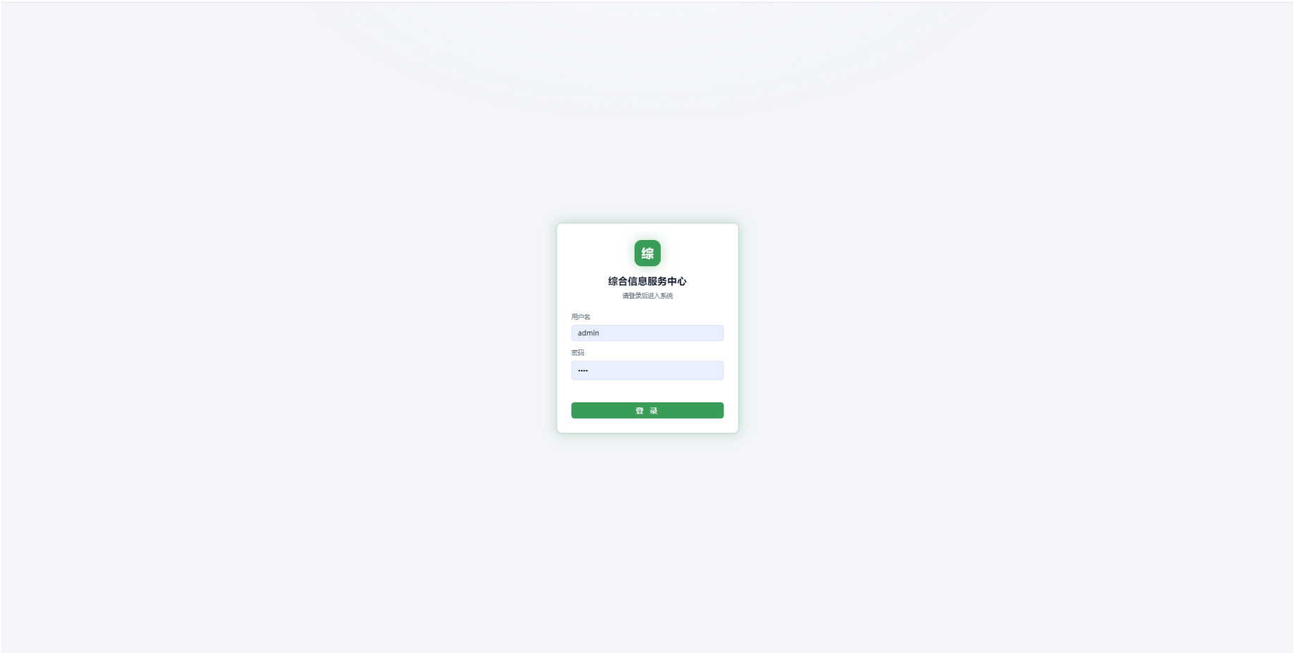
图 1 登录界面
