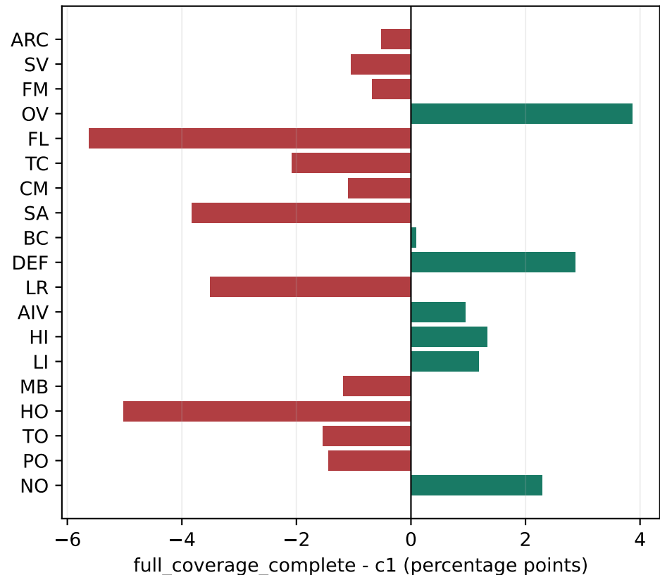
PR
