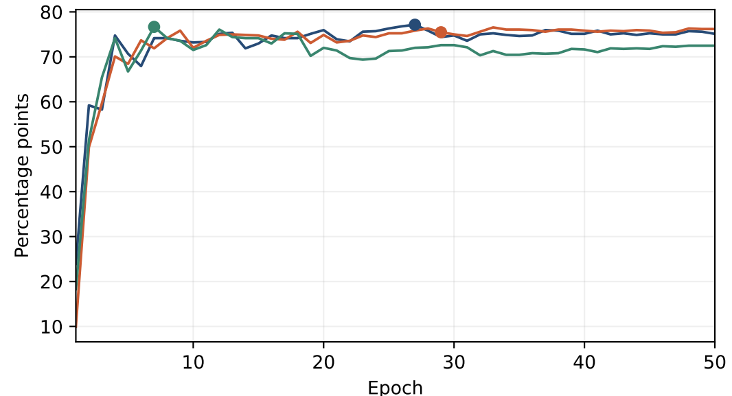
RGBNT100 — Rank-1
