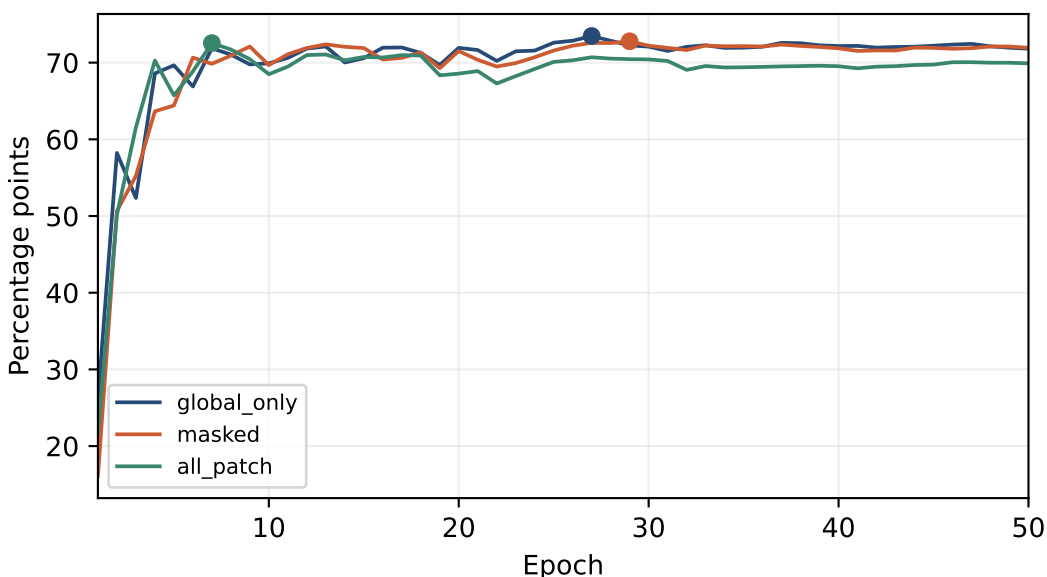
RGBNT100 — mAP
