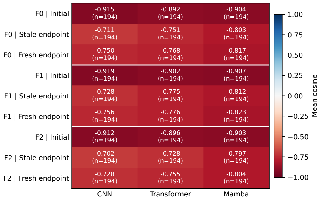
(d) Task total: \cos(G, G + \lambda g_V)
