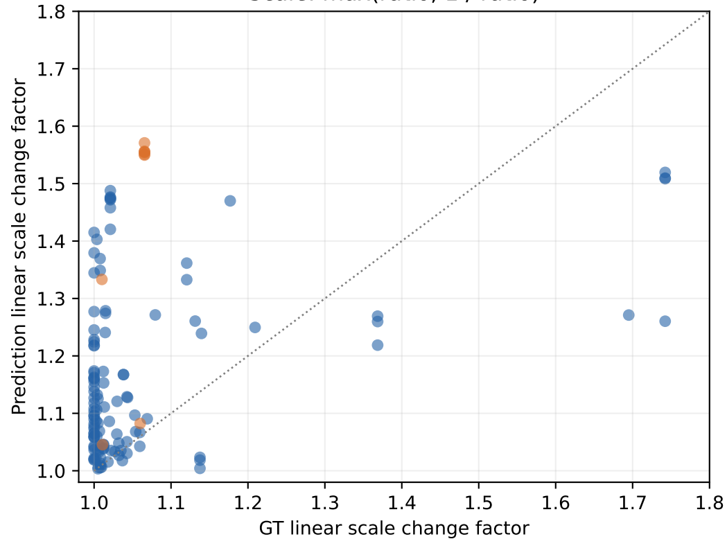
Scale: max(ratio, 1 / ratio)
