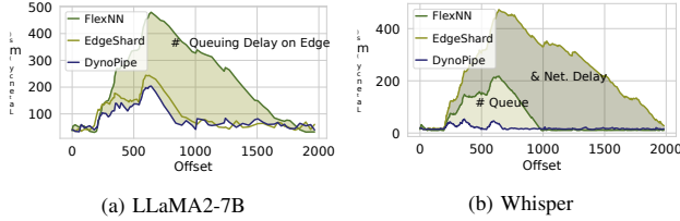
图 17: DynoPipe 和基线系统之间的延迟开销比较。开销是根据与专用 GPU 执行时间的差异来衡量的。(a) LLaMA2-7B。(b) 耳语。
