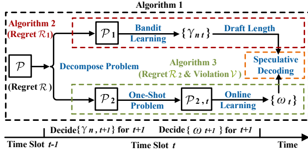
图 4: 理论分析路线图
