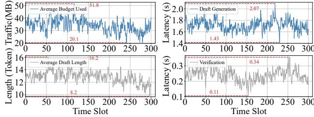
图 13: 盗匪学习
