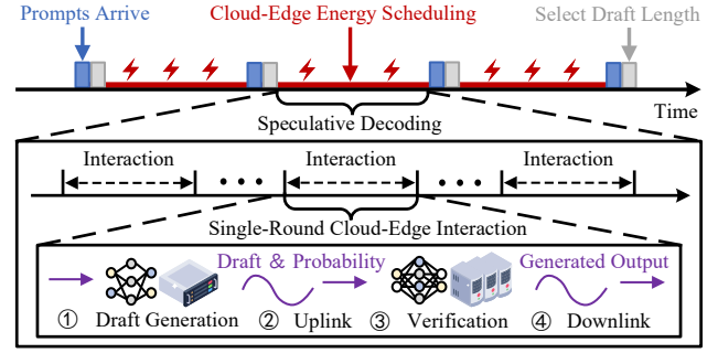
图 3: 云-边缘系统的时间流
