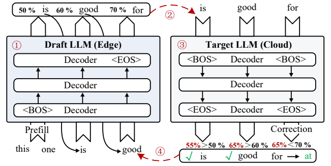
图 2: 投机解码的指示性示例: draftLLM 自回归生成草稿标记 is good for (步骤 1)，并将其发送到目标 LLM (步骤 2)；目标 LLM 验证并纠正它们 (步骤 3)，并将输出标记 is good at 返回给 draft LLM (步骤 4)。
