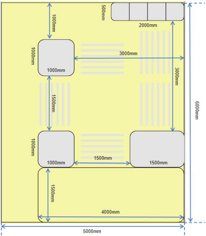
图 6-1 场地俯视图
