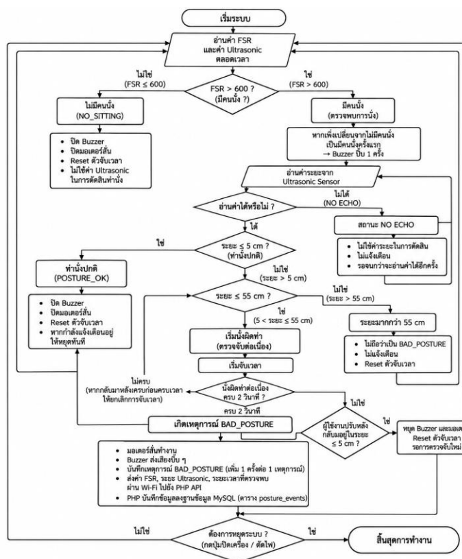
ภาพที่ 9 Flowchart ของ Shisei Kaizen ระบบแจ้งเตือนพฤติกรรมนั่งและช่วยปรับบุคลิกภาพ
