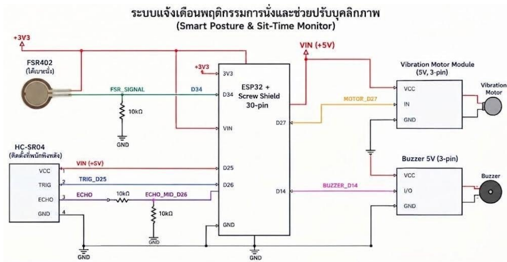
ภาพที่ 12 ไดอะแกรมวงจรไฟฟ้า (Schematic Diagram) ของ Shisei Kaizen ระบบแจ้งเตือนพฤติกรรมนั่งและช่วยปรับบุคลิกภาพ
