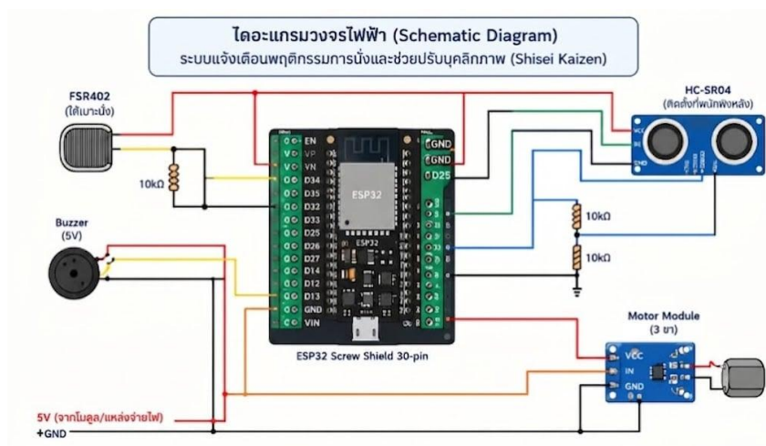
ภาพที่ 11 ไดอะแกรมการต่อสาย (Wiring Diagram) ของ Shisei Kaizen ระบบแจ้งเตือนพฤติกรรมนั่งและช่วยปรับบุคลิกภาพ
