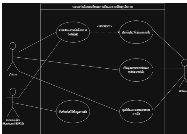
ภาพที่ 10 Usecase Diagram ของ Shisei Kaizen ระบบแจ้งเตือนพฤติกรรมนั่งและช่วยปรับบุคลิกภาพ
