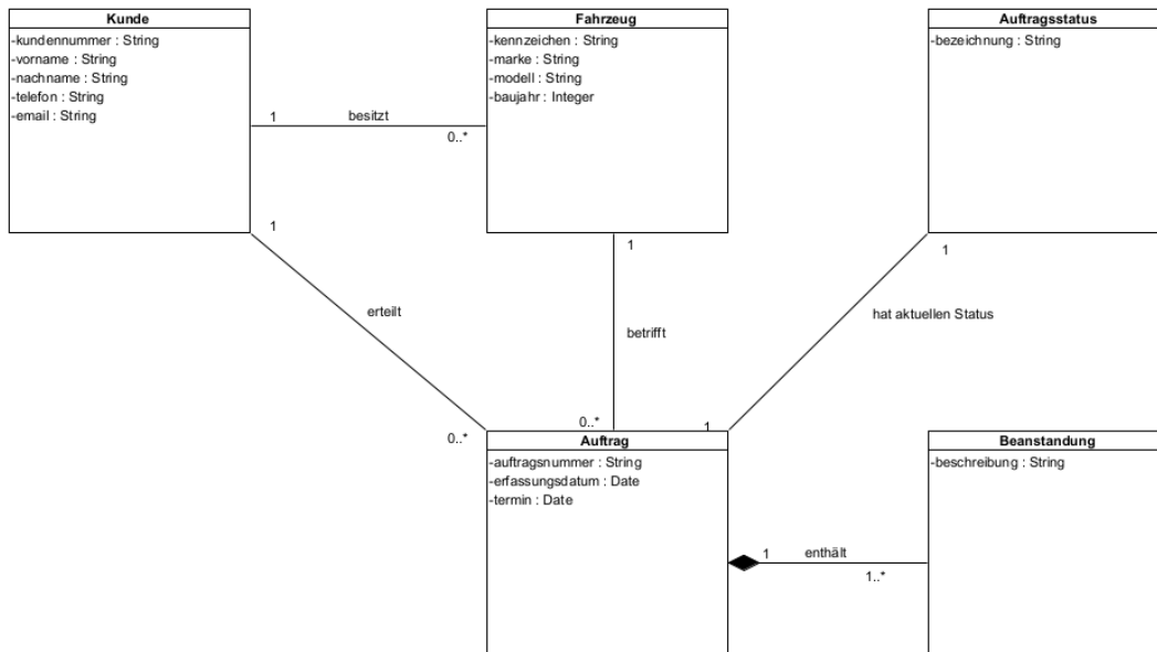
Abbildung 1: Fachklassenmodell WerkstattPilot, Iteration 1
