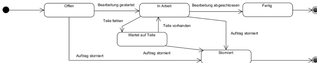
Abbildung 2: Zustandsmodell der Klasse Auftrag
