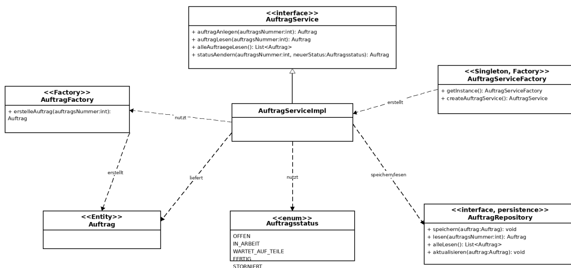
UML Klassendiagramm: Business-Schicht
