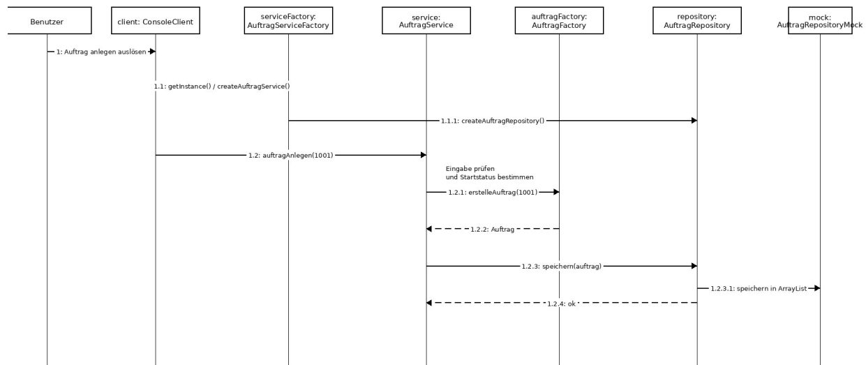
UML Sequenzdiagramm: UC1 Auftrag anlegen
