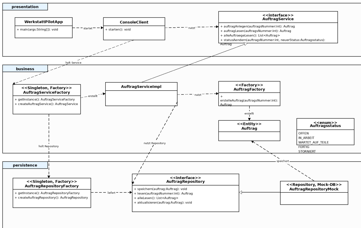
Abbildung 7: Aktualisiertes integriertes Klassendiagramm
