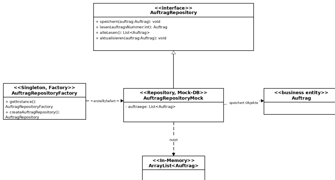
UML Klassendiagramm: Persistence-Schicht
