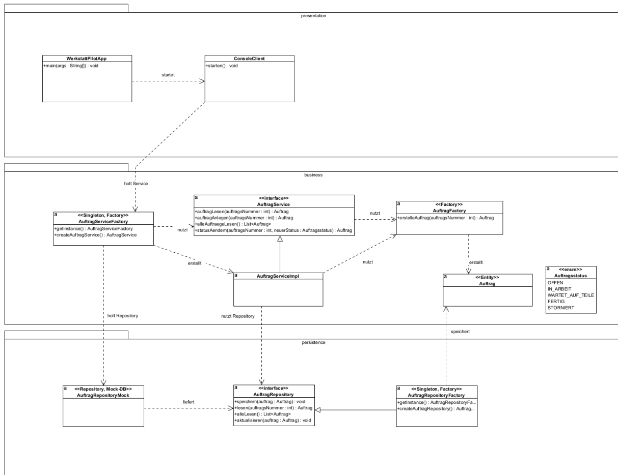
Abbildung 7: integriertes Klassendiagramm
