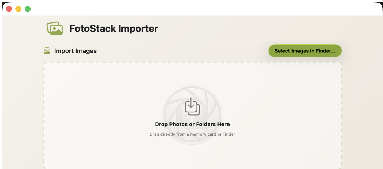
FotoStack Importer 1.0
