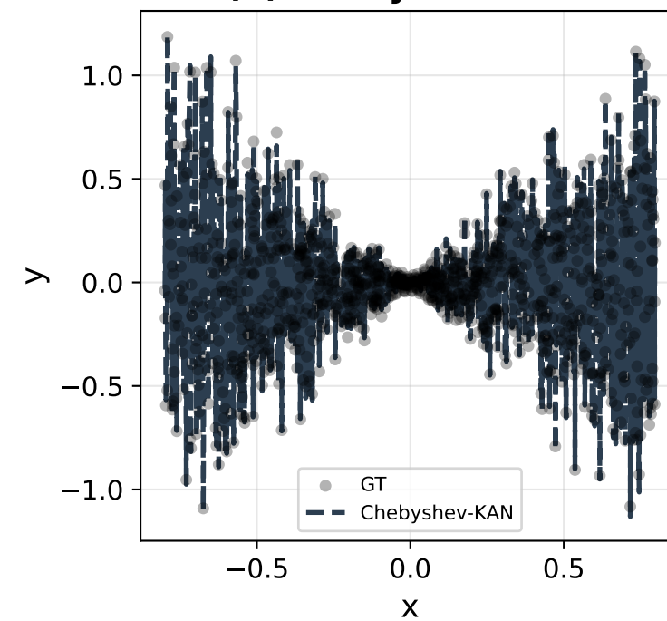
(h) Chebyshev-KAN
