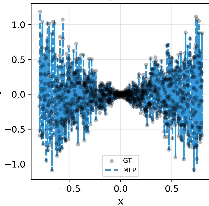
(e) MLP
