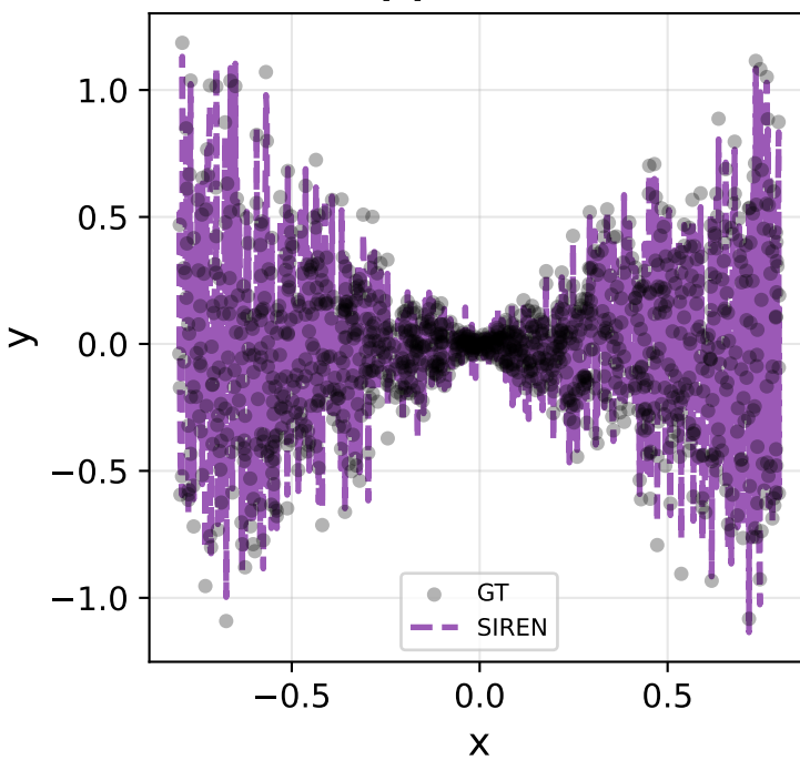
(f) SIREN
