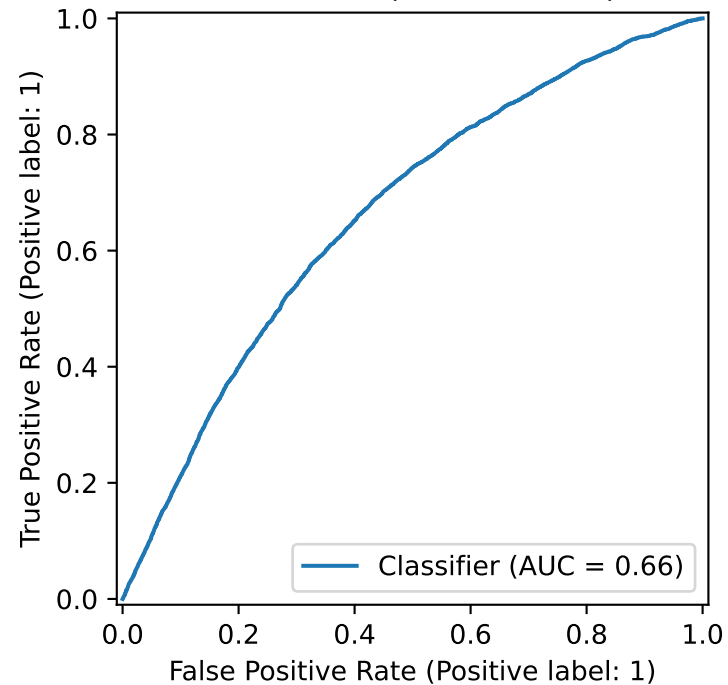
ROC curve (AUC = 0.664)
