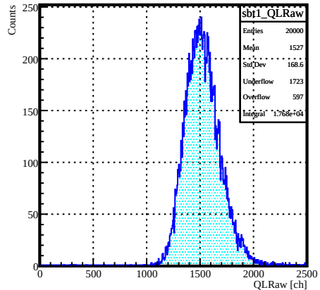
F13-1 / SBT1 QLRaw
