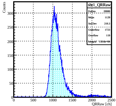
F13-1 / SBT1 QRRaw
