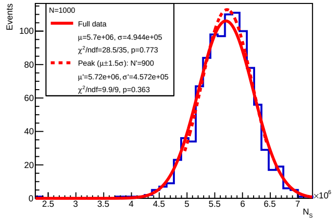
E = 40 GeV : N_S
