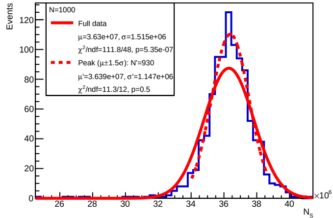
E = 250 GeV : N_S
