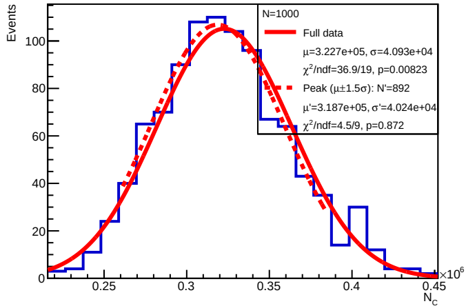
E = 250 GeV : N_C
