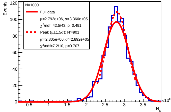
E = 20 GeV : N_S
