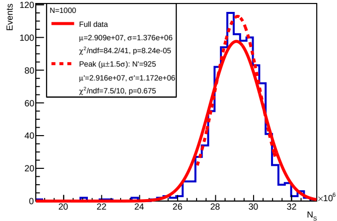
E = 200 GeV : N_S
