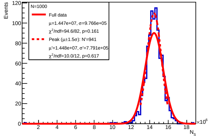
E = 100 GeV : N_S
