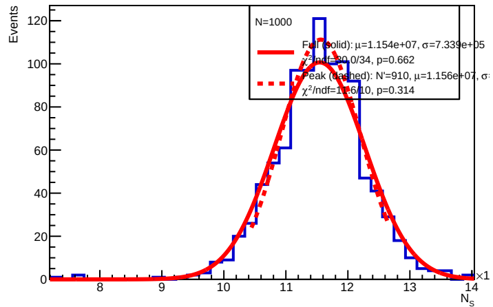
E = 80 GeV : N_S
