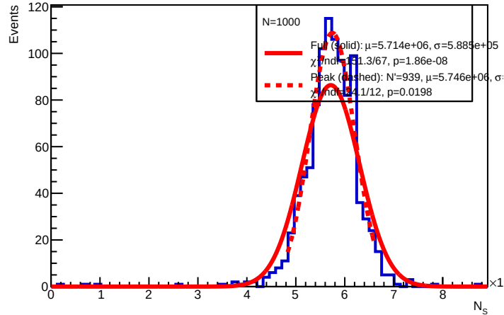
E = 40 GeV : N_S
