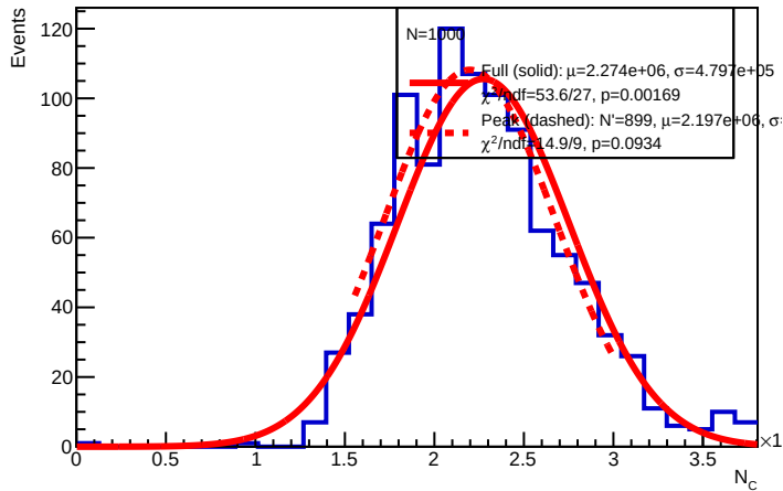
E = 100 GeV : N_C
