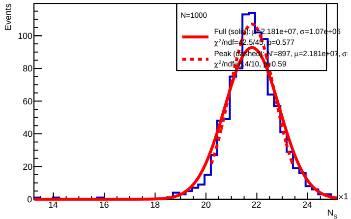
E = 150 GeV : N_S
