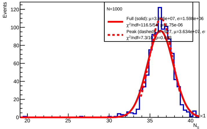
E = 250 GeV : N_S
