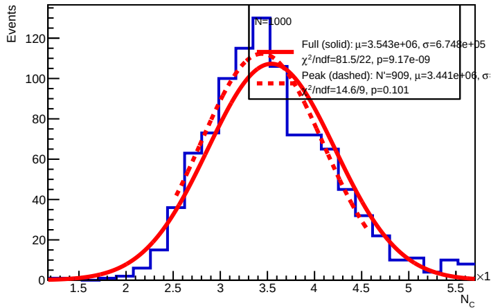
E = 150 GeV : N_C
