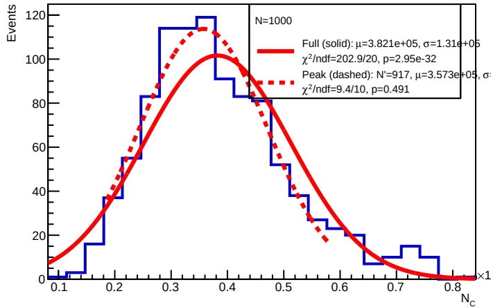
E = 20 GeV : N_C
