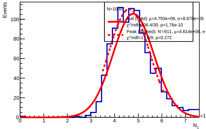
E = 200 GeV : N_C
