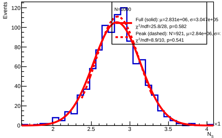
E = 20 GeV : N_S
