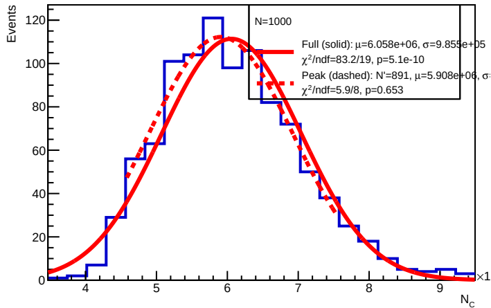
E = 250 GeV : N_C
