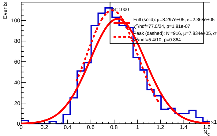
E = 40 GeV : N_C
