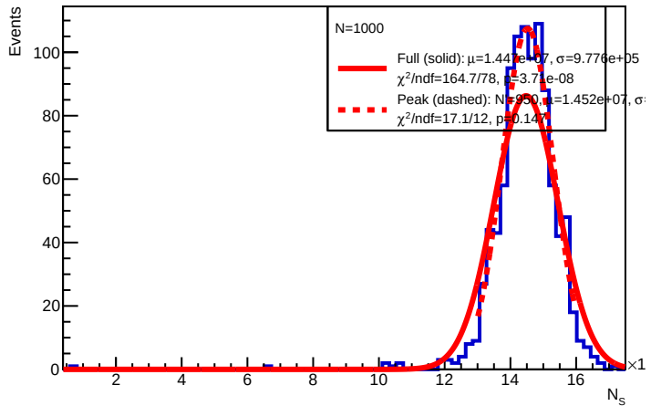
E = 100 GeV : N_S
