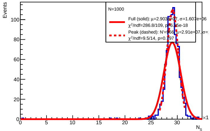
E = 200 GeV : N_S
