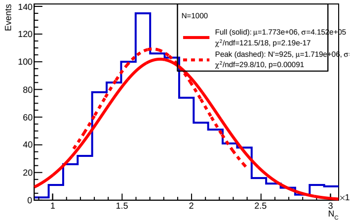
E = 80 GeV : N_C
