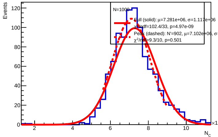
E = 300 GeV : N_C
