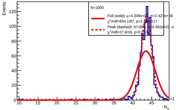
E = 300 GeV : N_S
