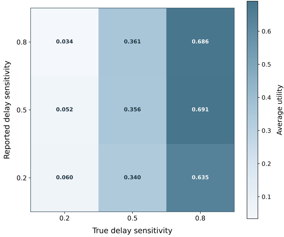
图 3: 不同真实时延敏感系数和申报敏感系数下的平均用户效用。
