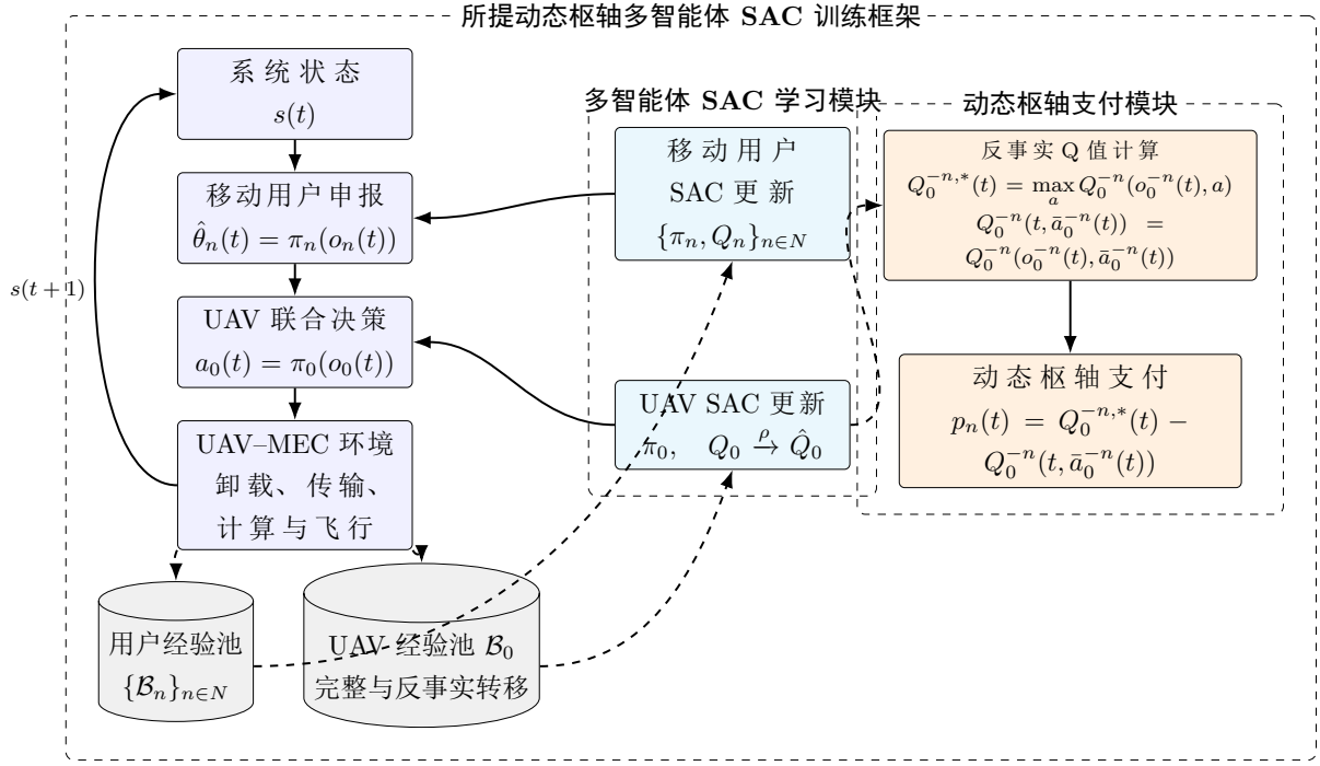
图 1: 基于动态枢轴机制的多智能体 SAC 框架。实线表示在线拍卖与环境交互，虚线表示经验采样、策略更新和反事实价值估计。
