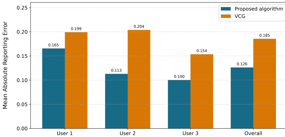
图 4: 所提方法与 VCG 基线下各用户的平均绝对申报误差。
