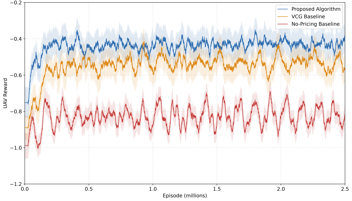
图 2: 所提方法与两类基线的 UAV 训练回报。阴影区域表示训练回报的波动范围。
