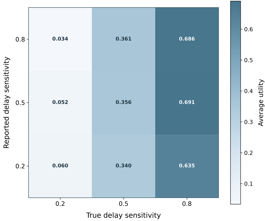
图 3: 不同真实时延敏感系数和上报敏感系数下的平均用户效用。
