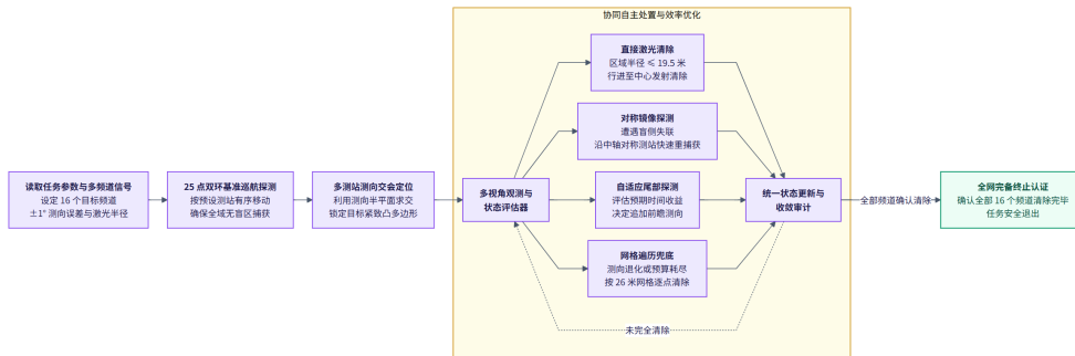
图 8 全向一定向混合干扰源自主协同搜索与清除系统架构图
