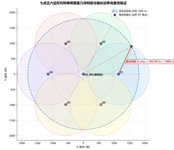
图 5 七点蜂窝全域覆盖几何验证
