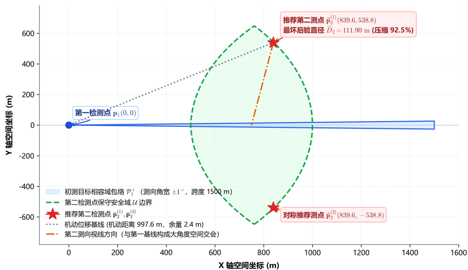
图3 第二检测点保守安全域 U 与推荐测点几何分布图
