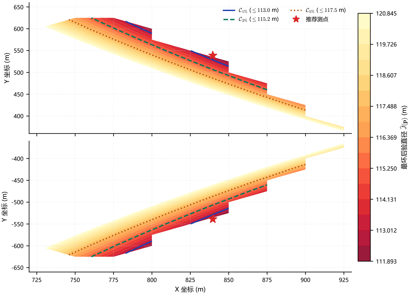
近优候选域 C_\tau 的双侧结构与目标等值线
